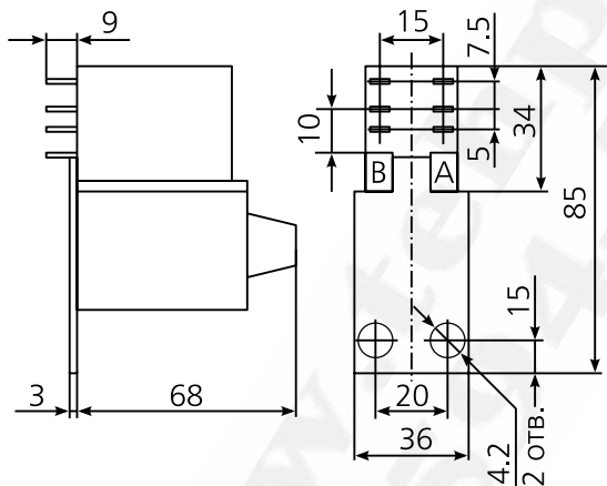
рис. 1 Крепление реле без розетки.
