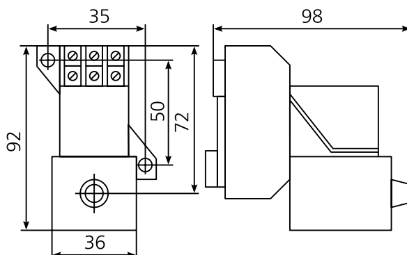
рис. 3 Крепление реле с розеткой типа 3.
